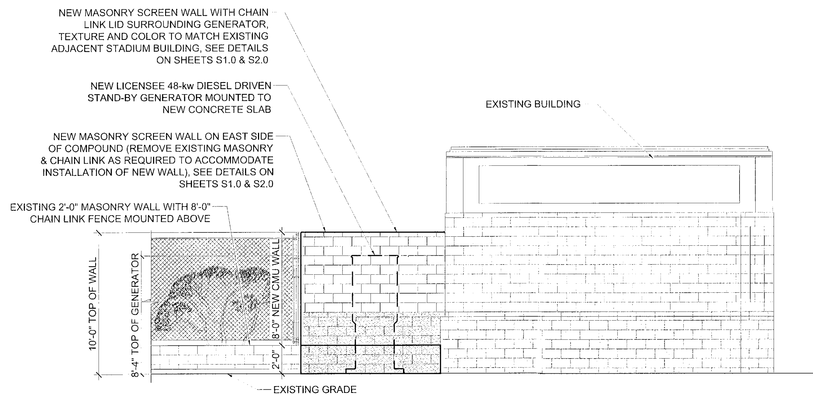
3 EAST GENERATOR ELEVATION A-3 SCALE: 1/4" = 1'-0"
