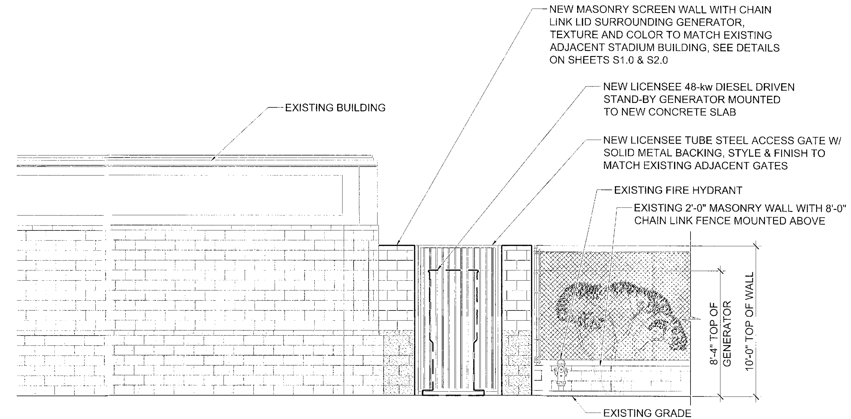
2 WEST GENERATOR ELEVATION A-3 SCALE: 1/4" = 1'-0"
