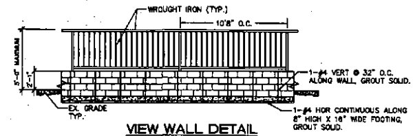
VIEW WALL DETAIL N.T.S.
