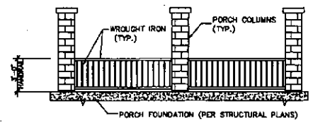
HAND RAIL DETAIL N.T.S.
