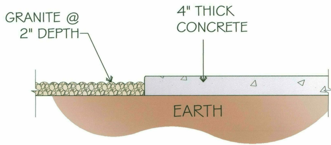
(D) CONCRETE DECK DETAIL
