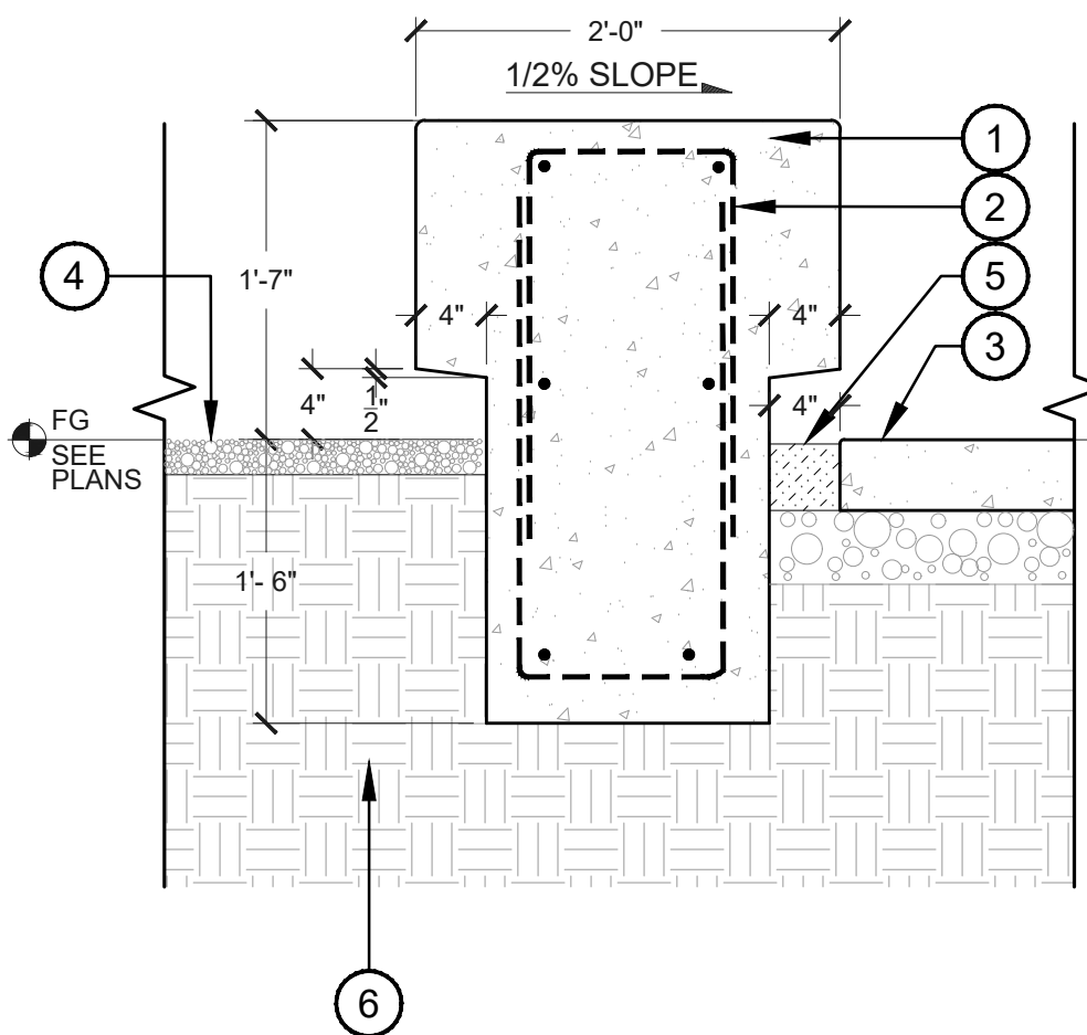
1 CIP SEATWALL SCALE: 1"=1'-0"
