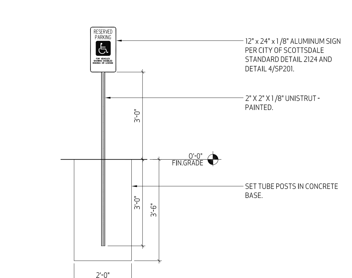
11 ACCESSIBLE SIGN (SCOTTSDALE) SCALE: 1/2"=1'-0"
