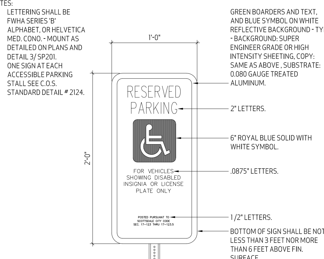
12 ACCESSIBLE SIGNAGE (SCOTTSDALE) SCALE: 1/2"=1'-0"
