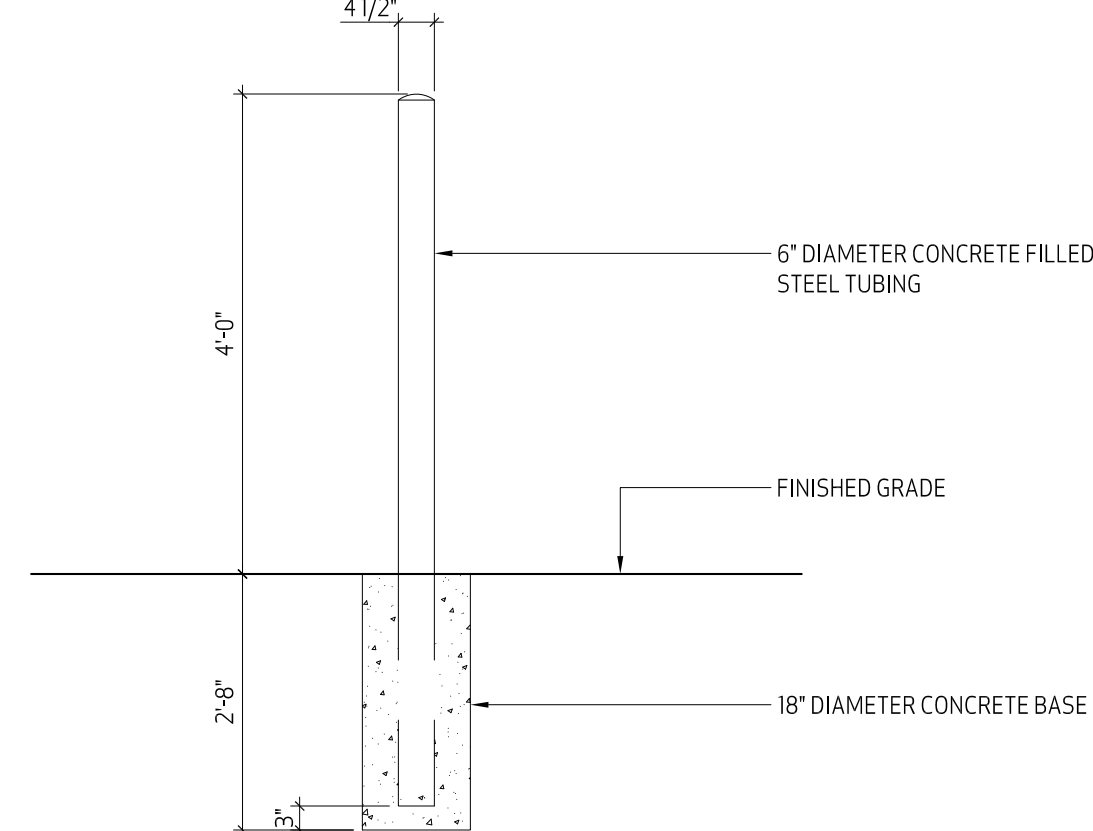
8 BOLLARD DETAIL SCALE: 1/2"=1'-0"
