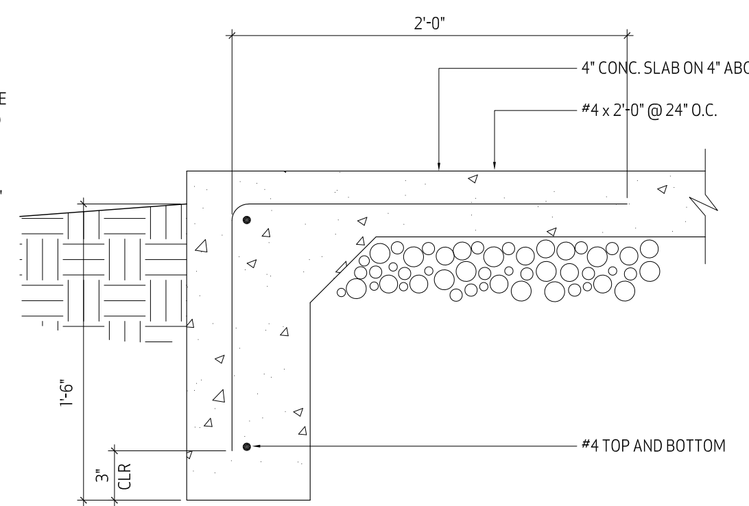
3 TURNDOWN AT SLAB EDGE
