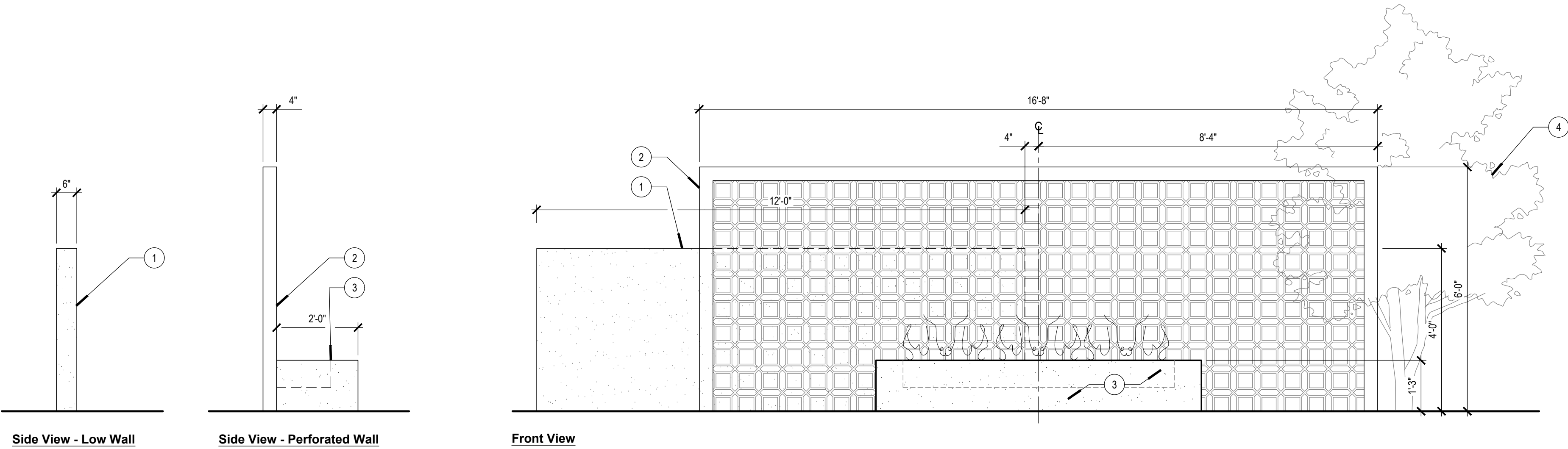
J Sonora Bloom Wall - Elevation Scale: 1/2" = 1'-0"
