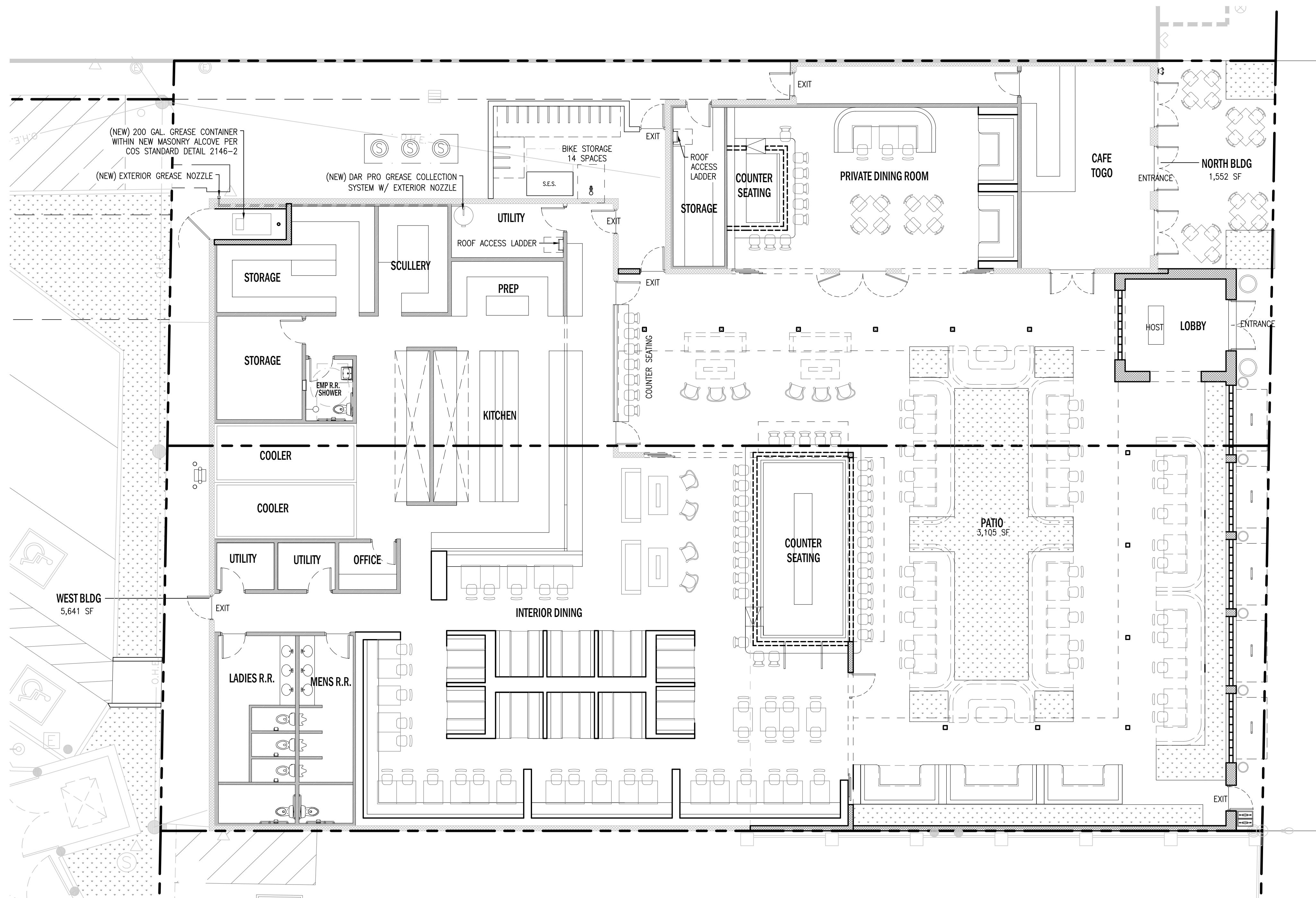
N FLOOR PLAN SCALE: 1/8" = 1'-0"
