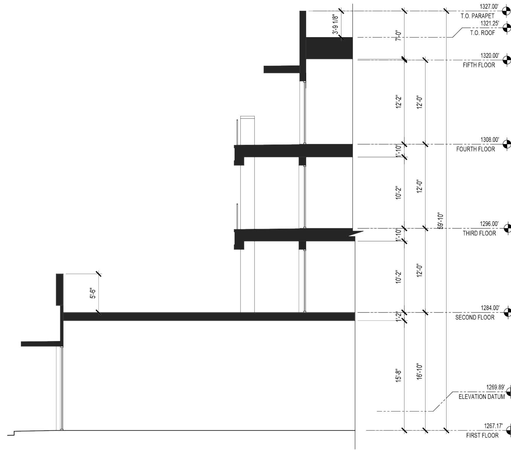
01 ENLARGEMENT A SCALE: 1/8"=1'
