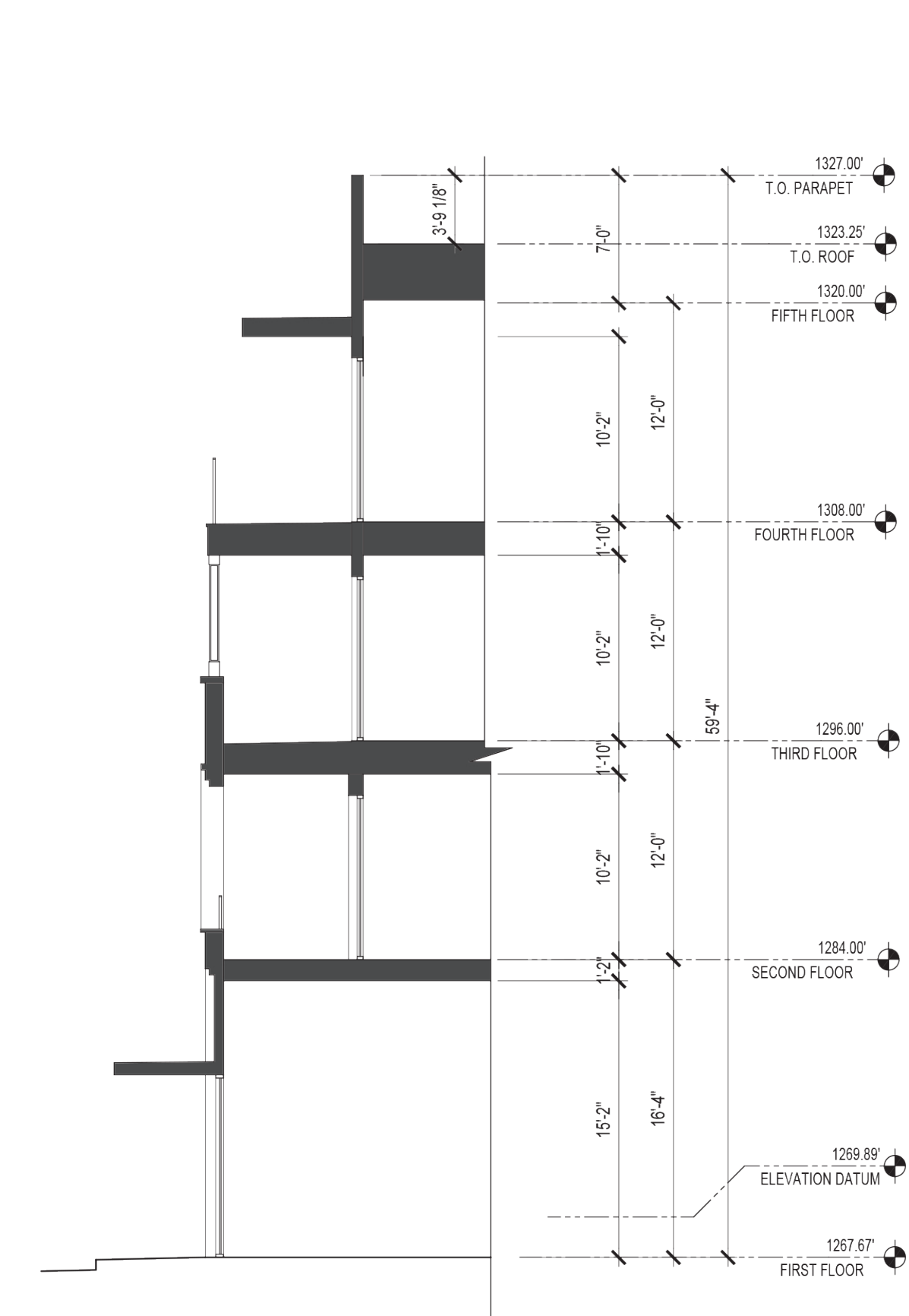
03 ENLARGEMENT C SCALE: 1/8"=1'
