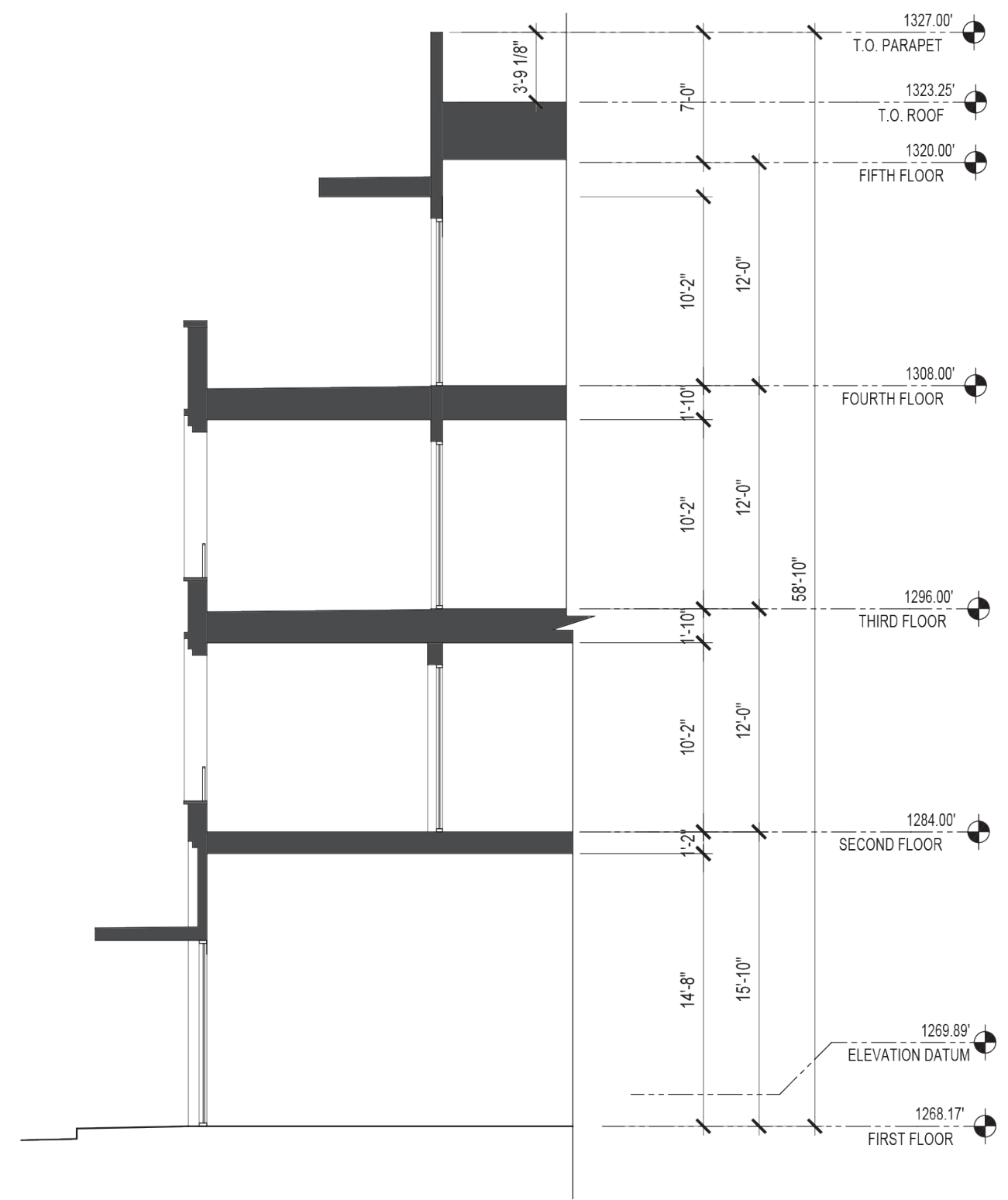
04 ENLARGEMENT D SCALE: 1/8"=1'
