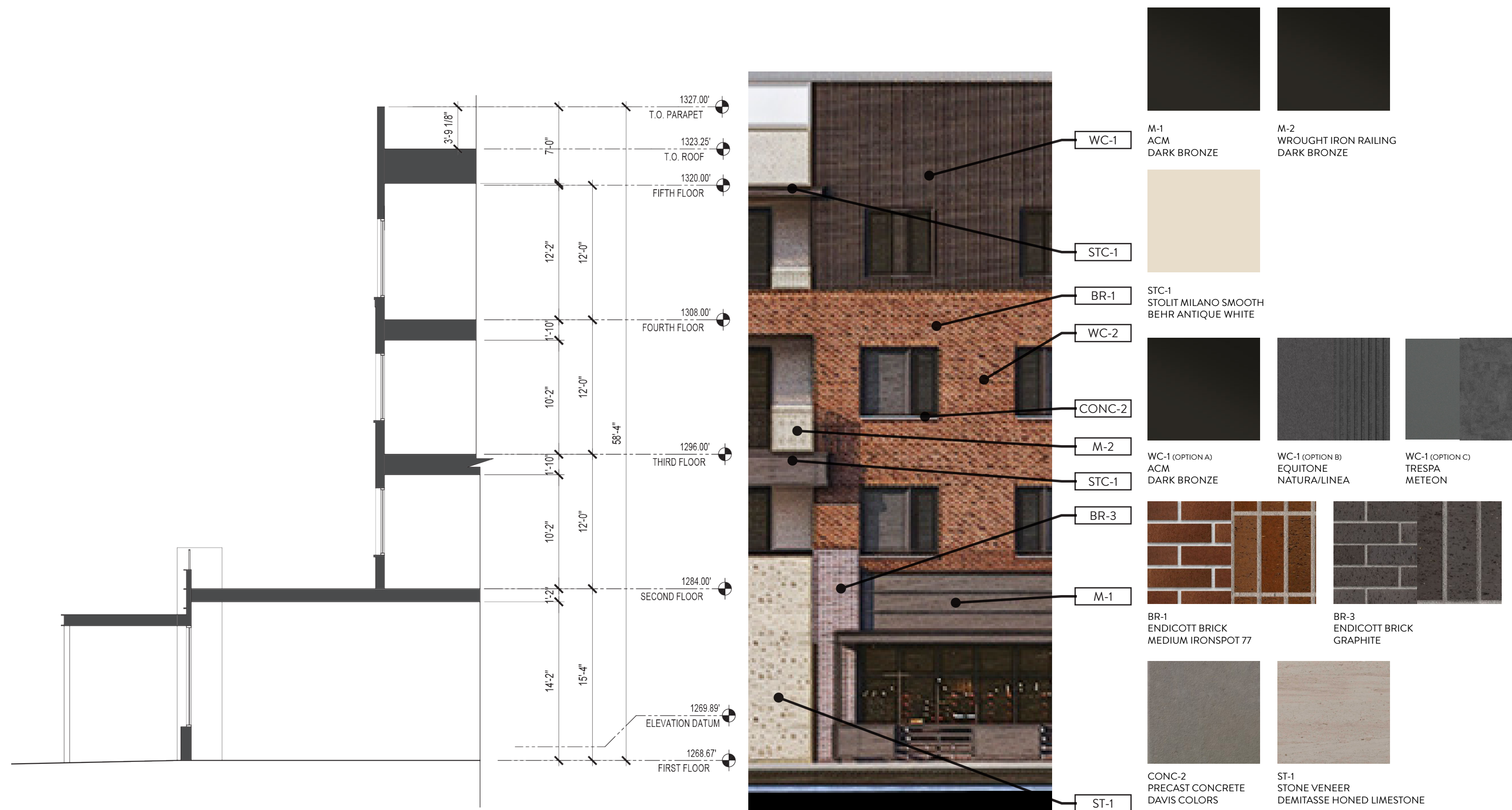
01 ENLARGEMENT E SCALE: 1/8"=1'
