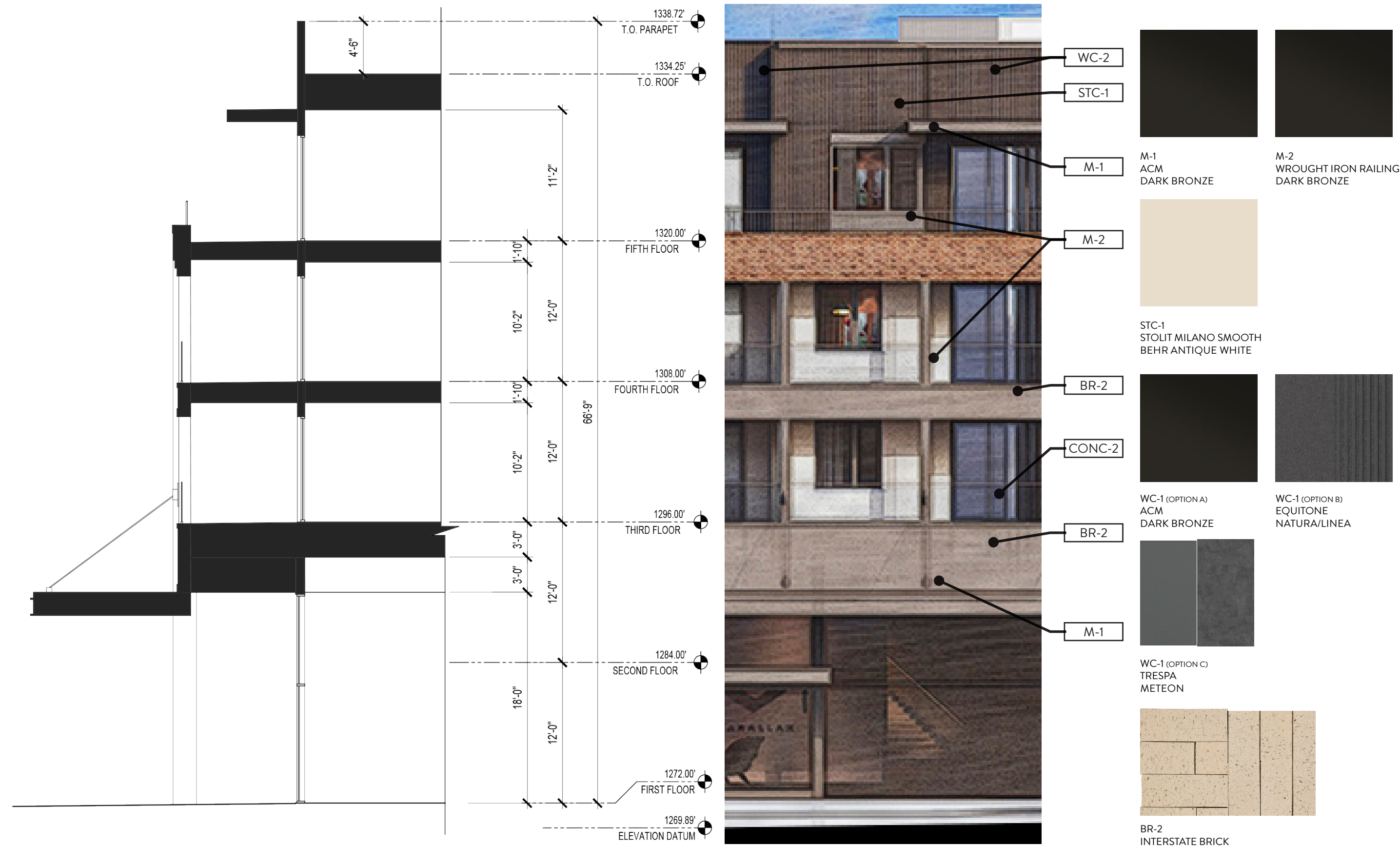
02 ENLARGEMENT F SCALE: 1/8"=1'
