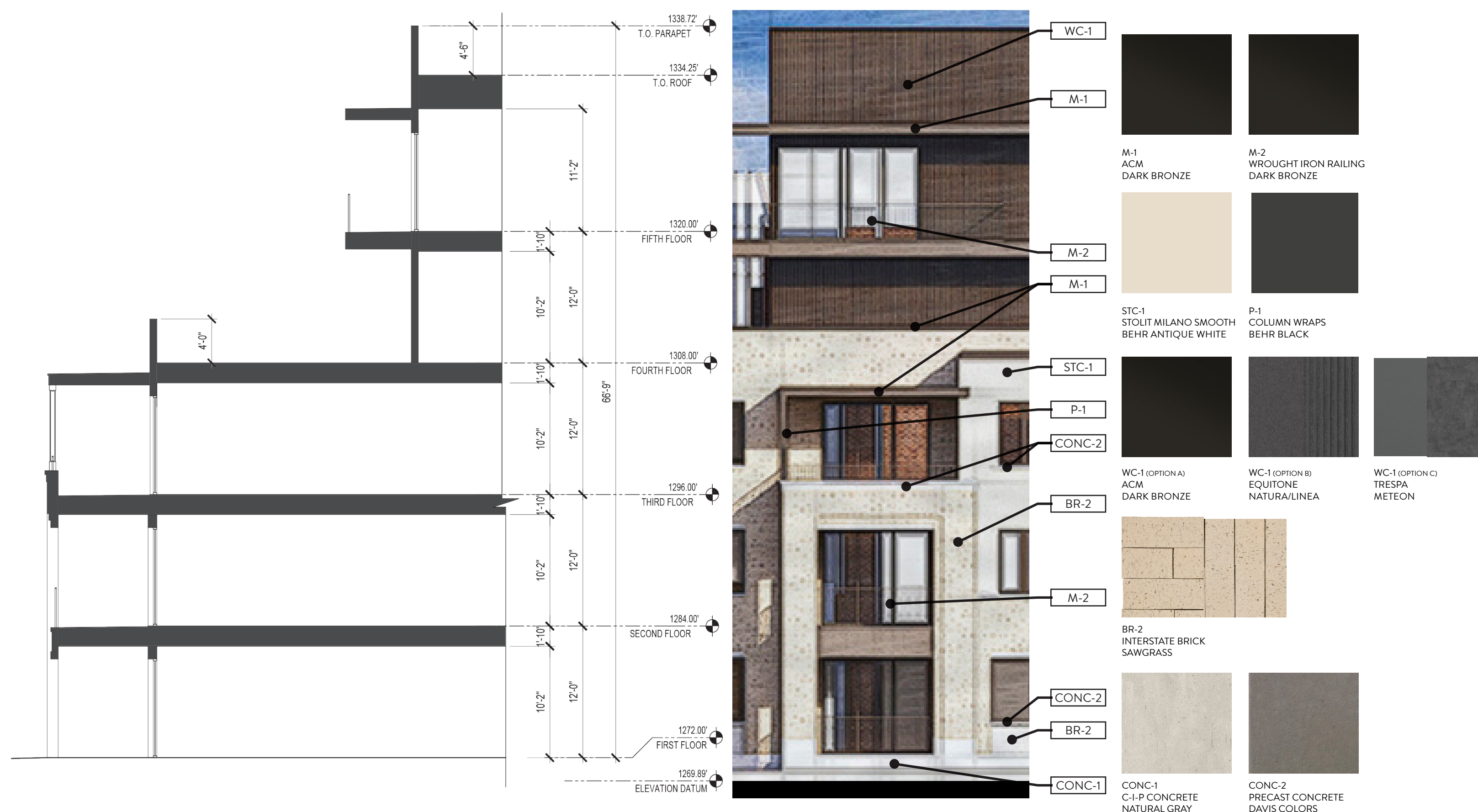
03 ENLARGEMENT G SCALE: 1/8"=1'
