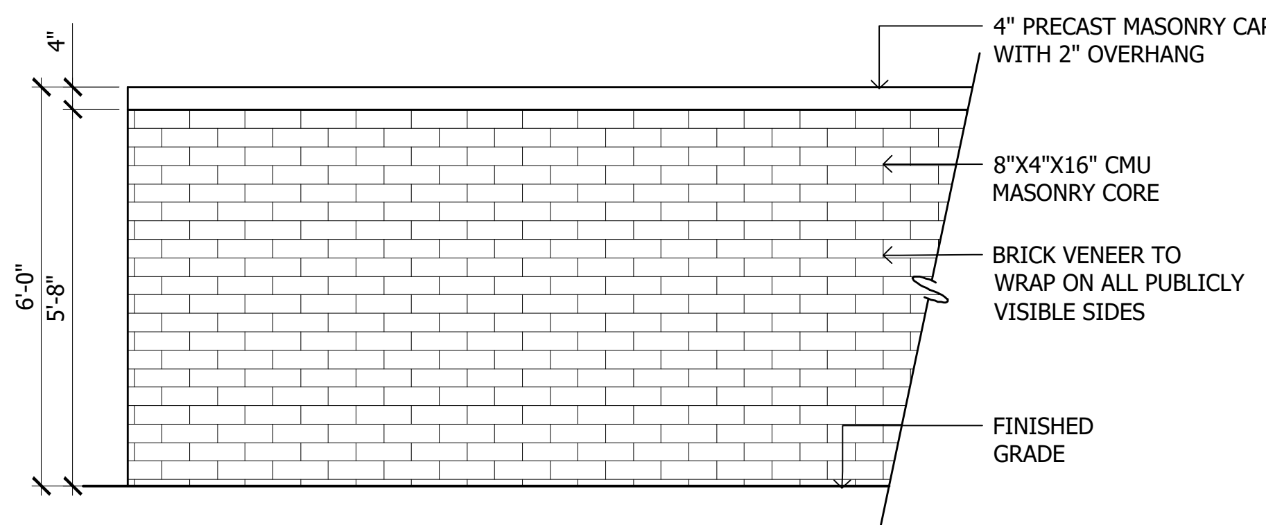
ELEVATION B
