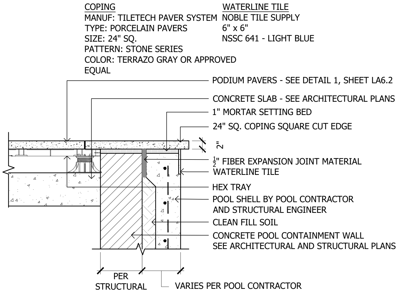
3 Pool & Spa Coping SCALE: 1"=1'-0"
