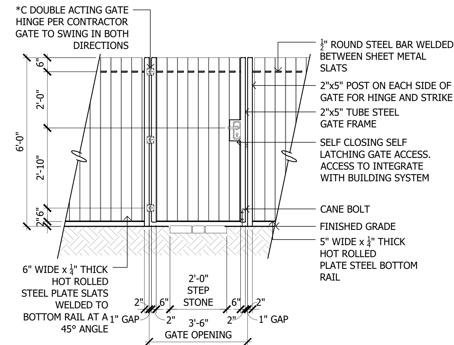
2 Slat Fence Gate SCALE: 1/2"=1'-0"
