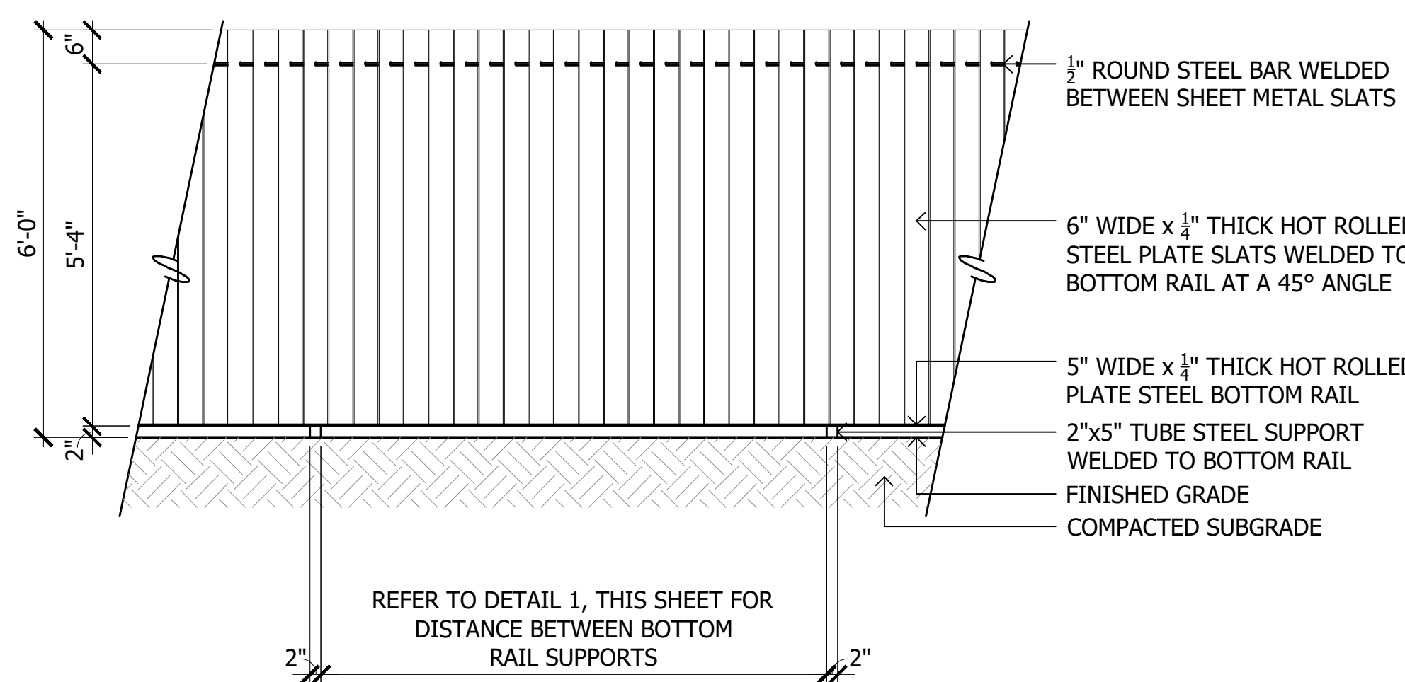
1 Slat Fence SCALE: 1/2"=1'-0"
