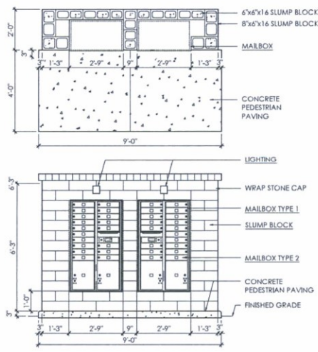
3 MAILBOX SCALE: 1/2" = 1'-0"
